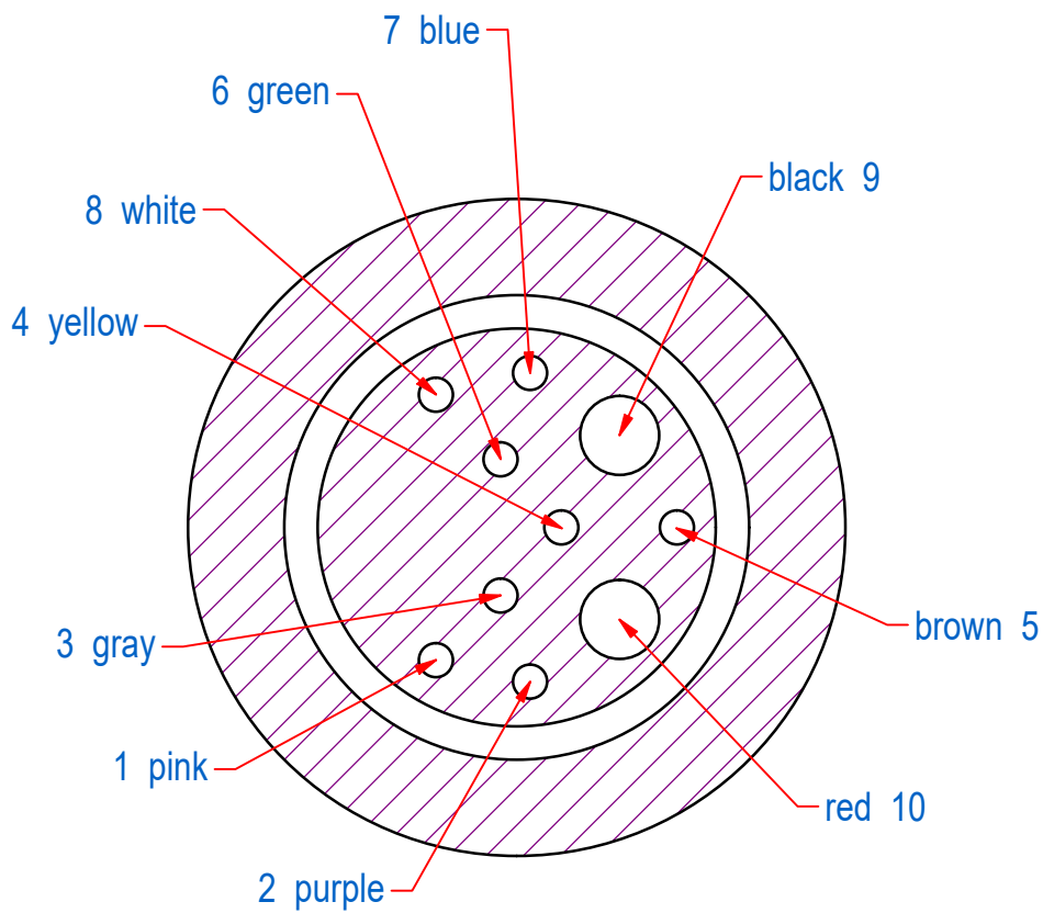
SECTION A-A ( 4 : 1 )
