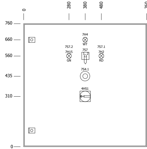
Voor-aanzicht
