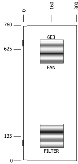
Zij-aanzicht
