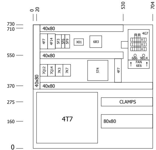
Montageplaat
