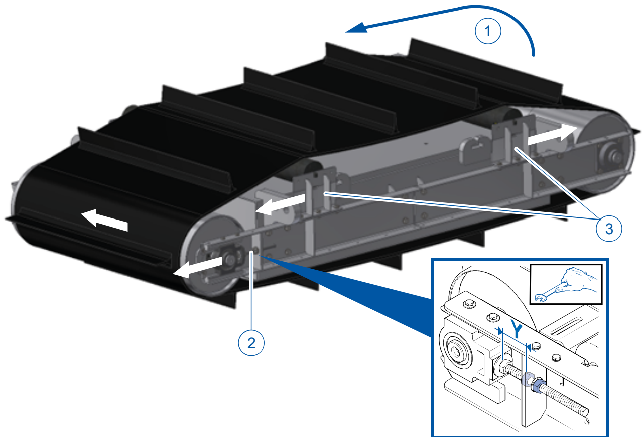
Afbeelding: Bandspanning afstellen
